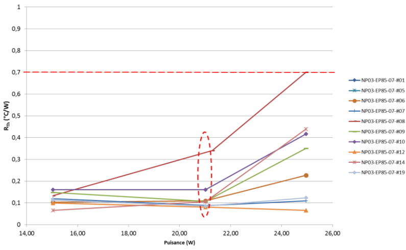
R_{Th}=f(P) - T_{condenseur}=25^{\circ}C - \text{Caloduc droit et étamé}
